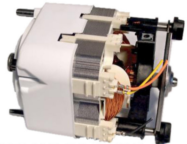
4573 MOTOR CUCINA Completa con Ventilador v Polea
